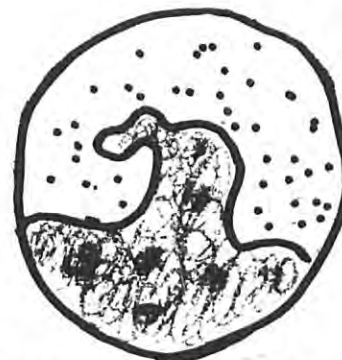
La nebulosa Cua de Cavall
