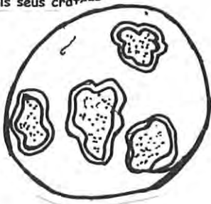
La Lluna amb els seus cràters
