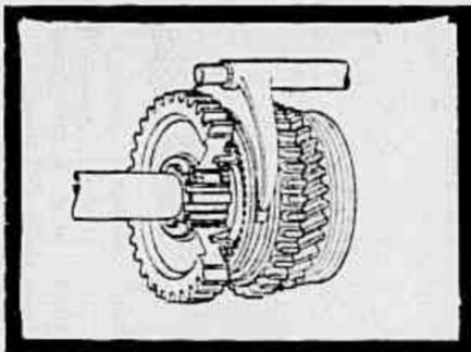
MAIOR RENDIMENTO — Caixa de câmbio com 5 marchas a frente (LP 321), todas sincronizadas, com reduções ideais, permite, em qualquer regime de marchas o aproveitamento ideal da economia do combustível e da força constante proporcionada pelo motor Mercedes-Benz Diesel, dispensando as reduções especiais no diferencial e assegurando maior rendimento.
