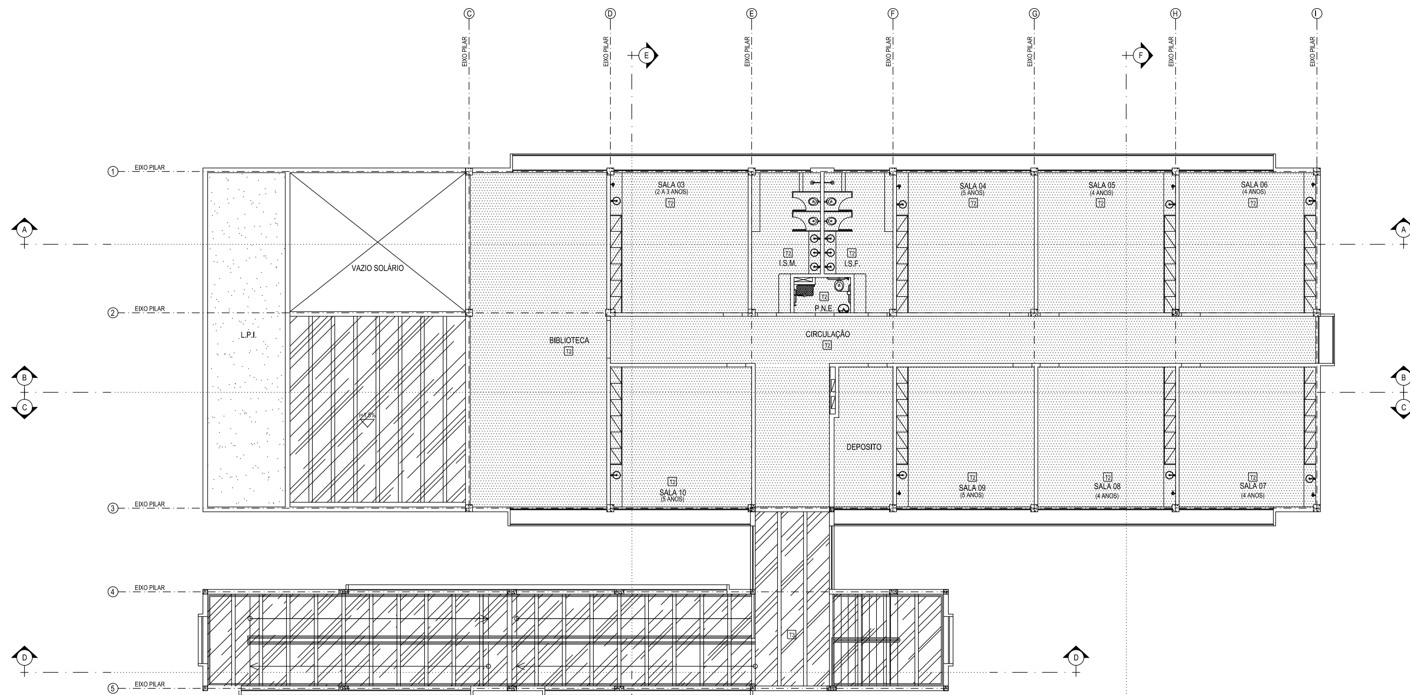
UMEI KENNEDY PLANTA DE FORRO 3º PAVIMENTO ESCALA: 1/100
